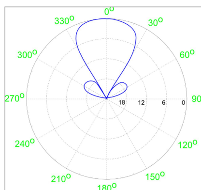
Vyzářovací diagram ve V-rovině
