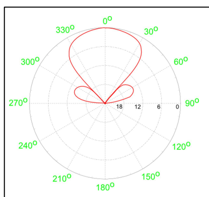
Vyzářovací diagram v H-rovině
